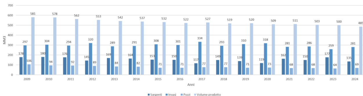
PRELIEVO IDRICO DI ACQUEDOTTO PUGLIESE PER TIPOLOGIA DI FONTI
